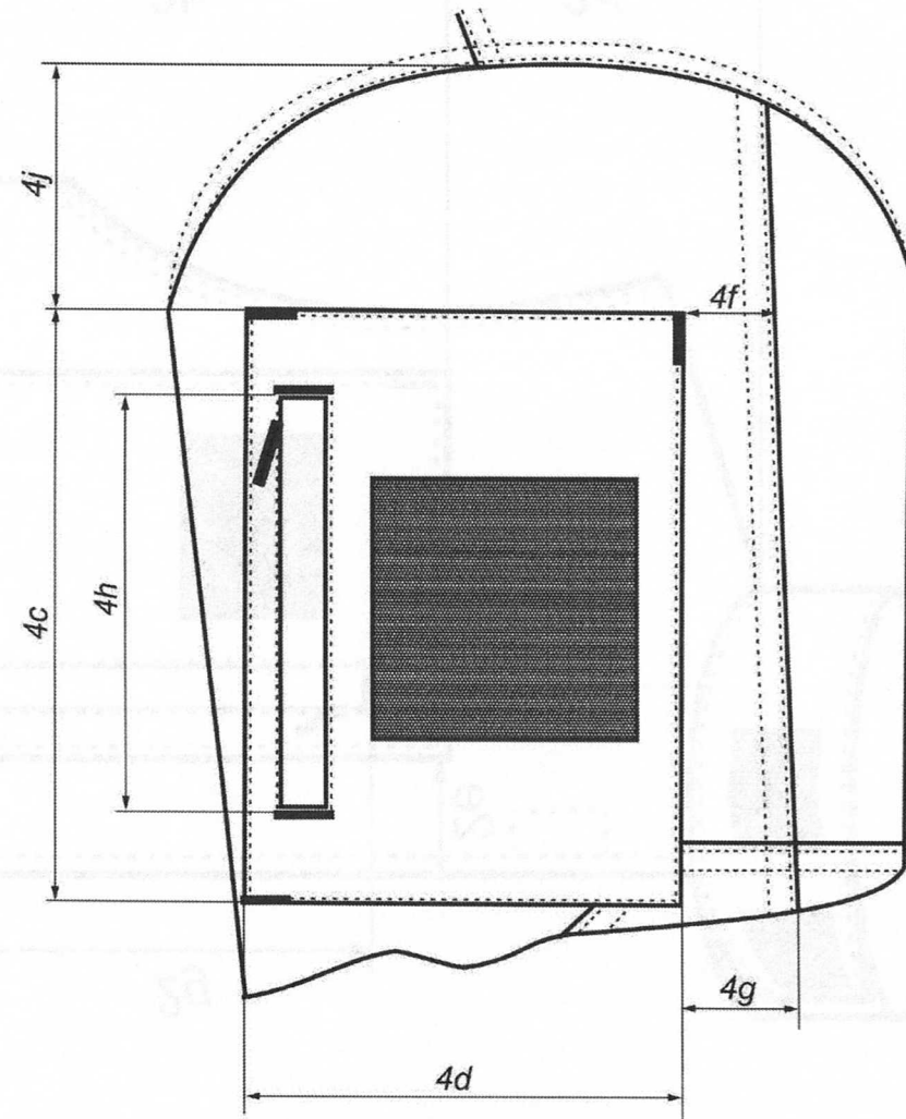
Rysunek 4 – Kieszka gorna rękawa
